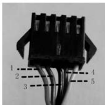
Zapojení displeje
